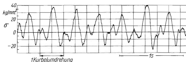
Bild 24. Spannungen in einem Heuwenderzinken [12].
