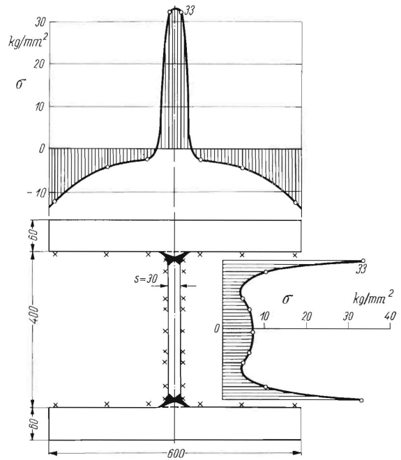
Bild 11. Eigenspannung durch Schweißung eines I-Trägers nach Bierett [6].
