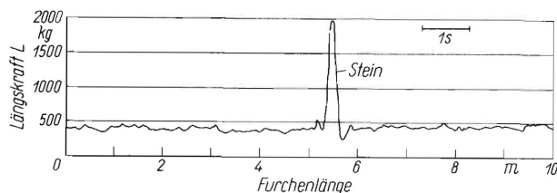
Bild 23. Stör- und Betriebskräfte in Fahrtrichtung am Pflug [11].
