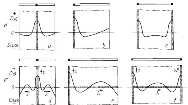
Bild 12. Eigenspannungen nach dem Schweißen nach Bierett [6].
